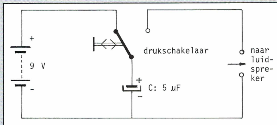
Fig. 8. Schema van het pulsertje voor effectieve luidsprekerbeoordeling.
