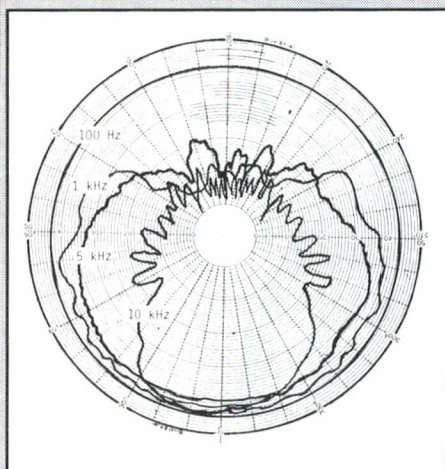
Fig. 1. Rondstraalkarakteristiek van een tweewegsysteem. Hoe hogere frequentie, hoe gerichter de weergave.
